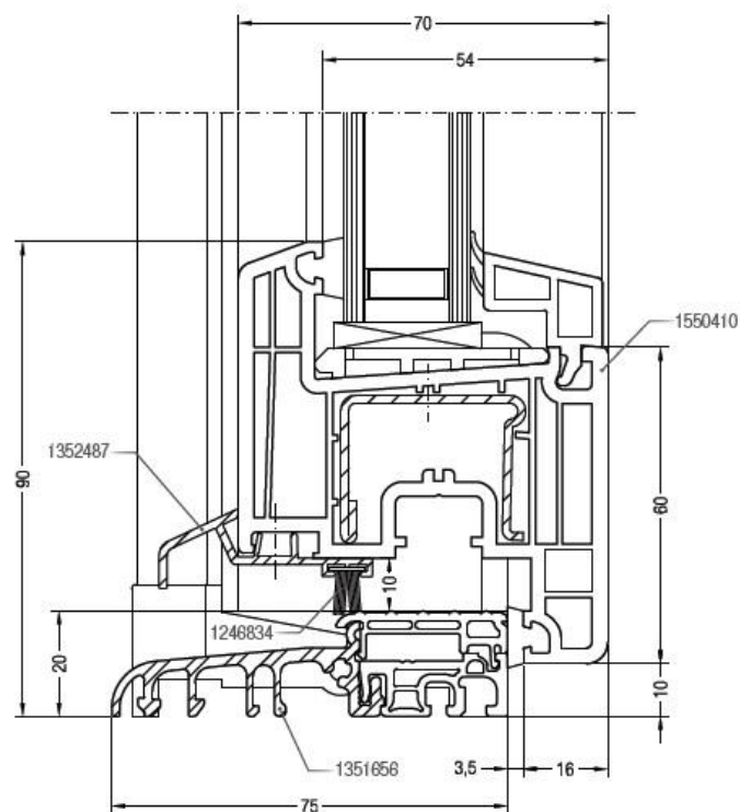
Sezione nodo anta dritta da 60 mm e soglia in Al Brillant 70
